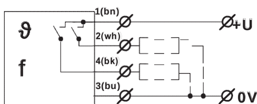
Zapojení průtokoměru ETDF-25
