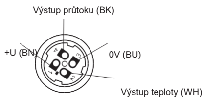
Vnitřní pohled na konektorovou zásuvku (varianta "C")
