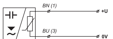
Zapojení snímače s výstupem typu NAMUR (provedení Xi, XiM, XiT, XiMT)
