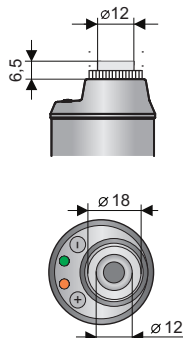
Provedení „C“ s konektorem M12
