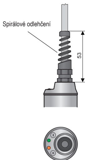
Provedení „V“ s plastovou vývodkou se spirálovým odlehčením - pro případ zvýšeného mechanického namáhání kabelu.
