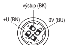
Vnitřní pohled na konektorovou zásuvku
