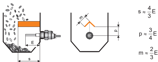
Montáž ochranné stříšky
