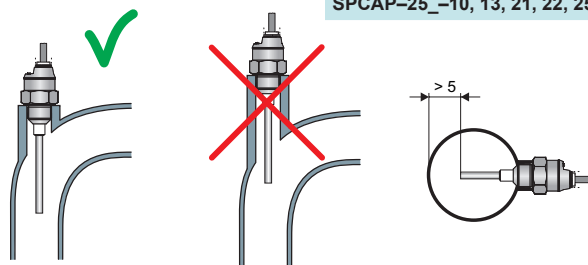
Montáž snímače do trubky
